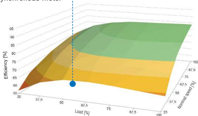
IE3 asynchronous motor
